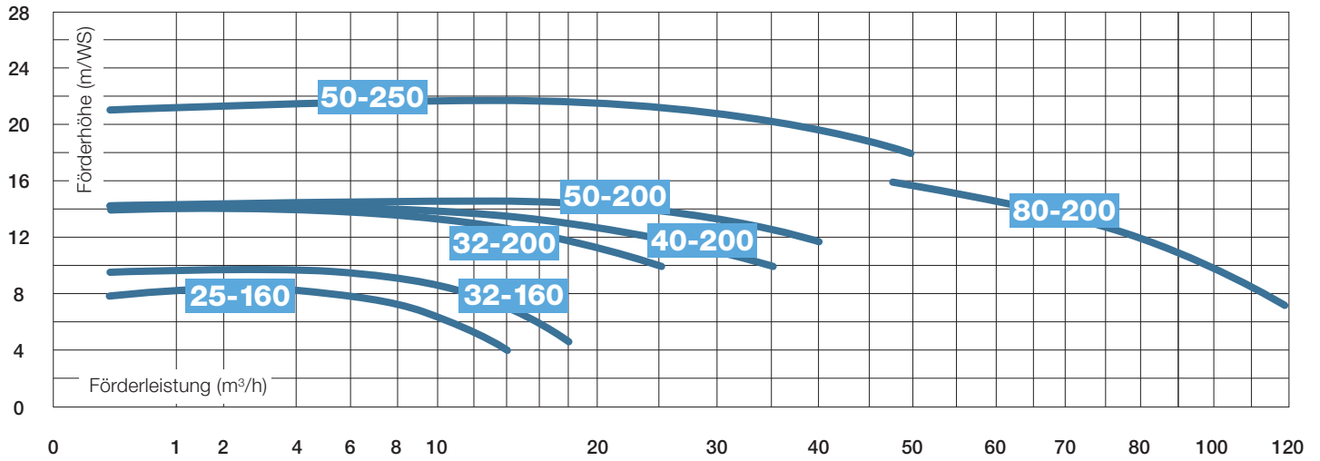
Kennlinie NM ( n = 2900 \text{ min}^{-1} , 50 Hz)
